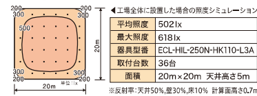
縫製工場
